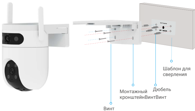
Рисунок 2. Монтаж на стену
