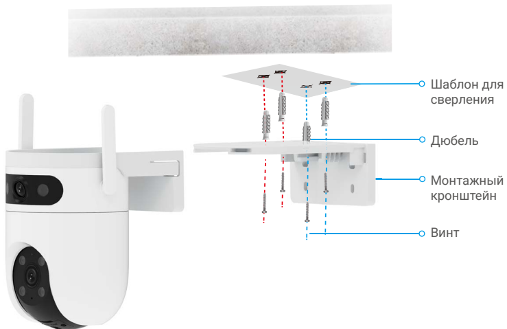
Рисунок 1. Монтаж на потолок
